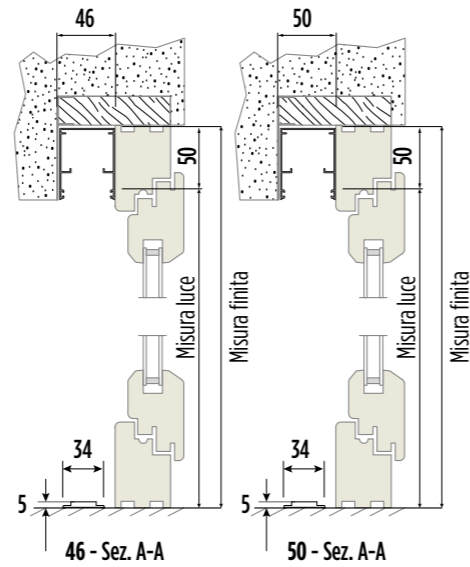
SEZIONE VERTICALE VERTICAL SECTION
