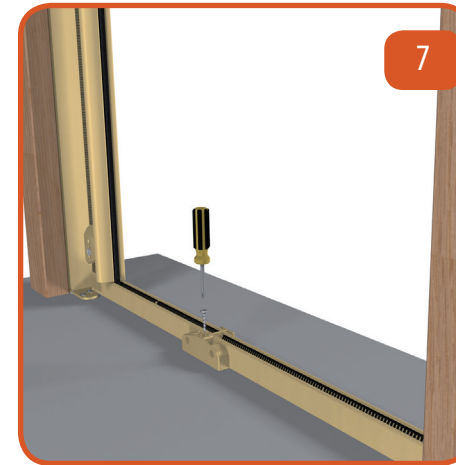
7 Posizionare al centro e fissare con le viti il reggi guide inferiori.
