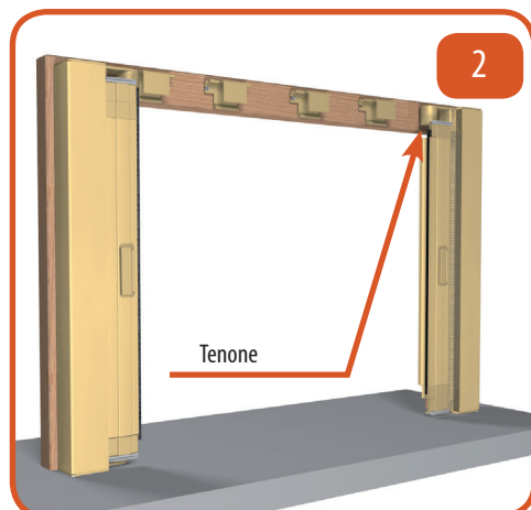
2 Posizionare i cassonetti con le testate con i tenoni verso l'alto.
