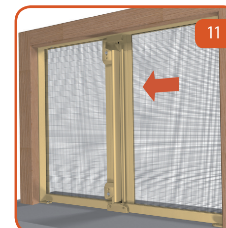
11 Applicare (se non già montate) le maniglie pieghevoli esterne. Collaudare la zanzariera.
