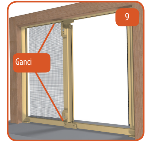
9 Regolare i ganci della barra maniglia semi fissa in modo che alzandola si sganci.
