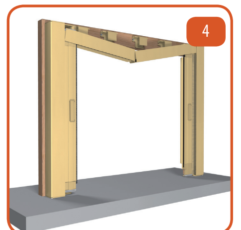
4 Posizionare le guide superiori facendole scattare nei supporti reggi guida.
