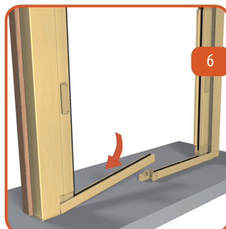
6 Posizionare le guide inferiori infilandole nelle alette delle testate.
