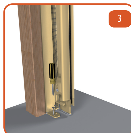
3 Fissare con le viti i cassonetti a terra.
