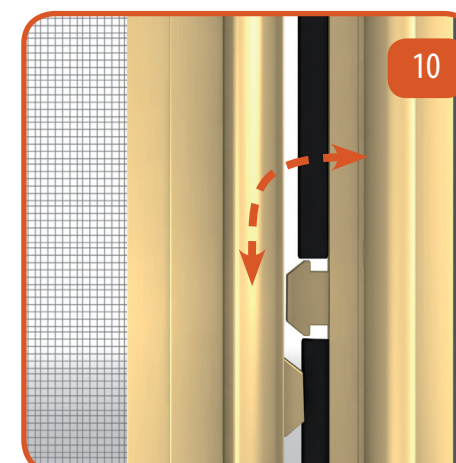
10 Regolare i ganci all'interno della barra maniglia grande in modo che alzando quella più piccola si sganci.
